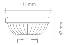
QLAMP 111 - AR111
